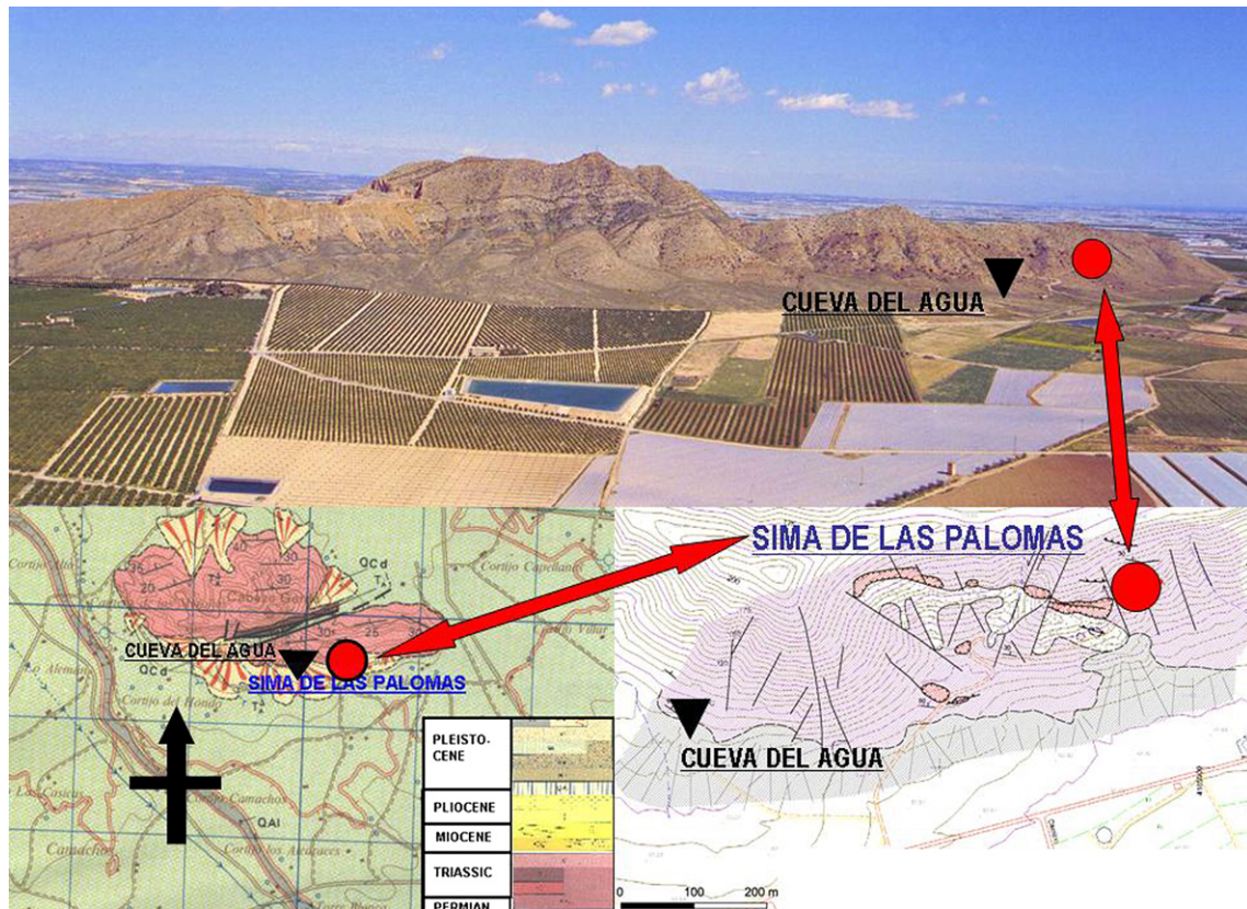
Fig. 2. Cabezo Gordo showing Sima de las Palomas, Cueva del Agua, and local geology.
